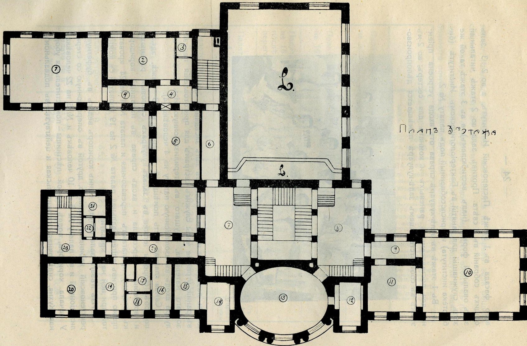
Планъ 3-го этажа, гдѣ преимущественно размѣщенъ Лазаретъ № 4.
